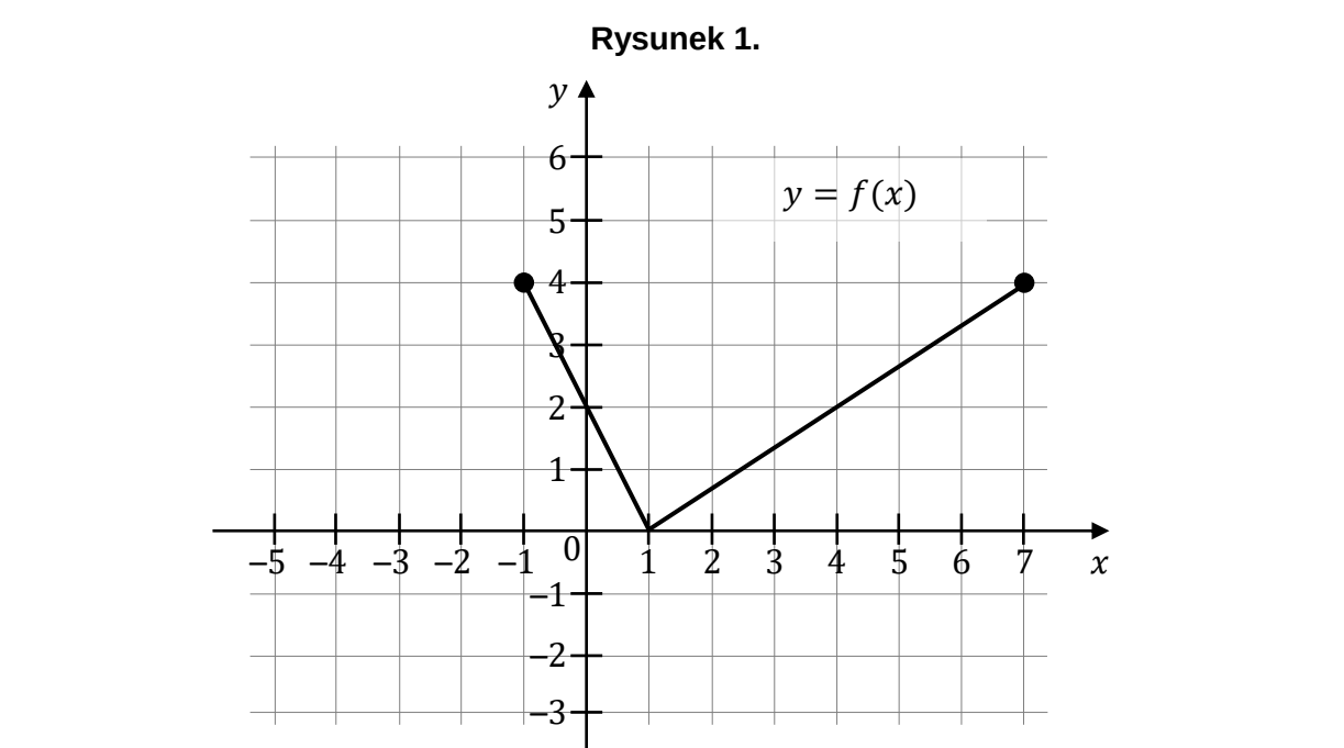
Na rysunku 1., w układzie współrzędnych (x, y) , przedstawiono wykres funkcji f .
